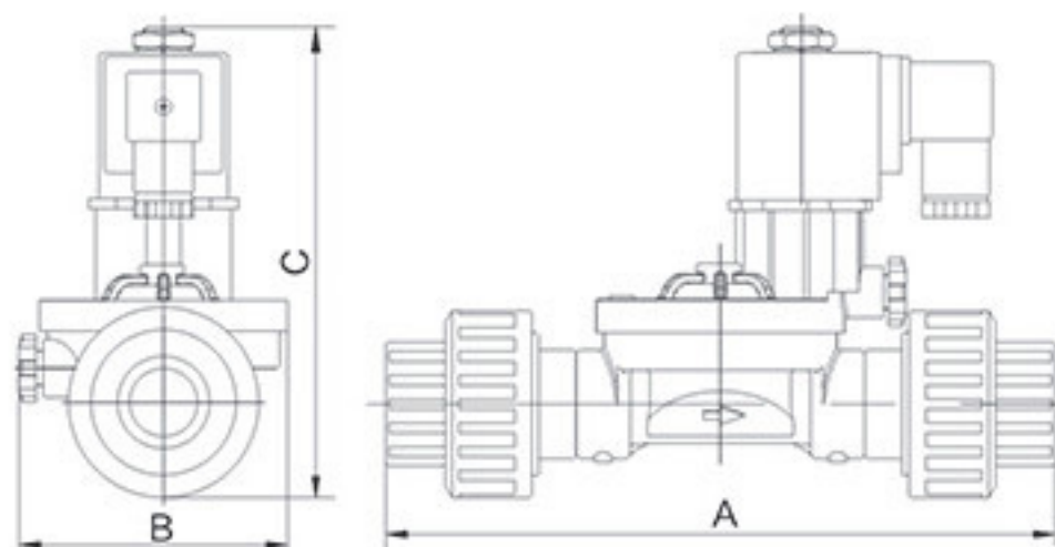
活接式外形图 (配DIN43650A接线盒)
