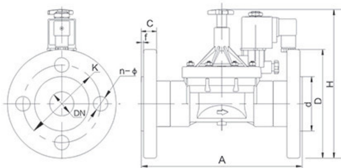
法兰式外形图 (配DIN43650A接线盒)
