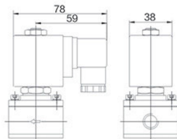
UZCF系列（常闭型）电磁阀外形结构图 （配DIN43650A接线盒）
