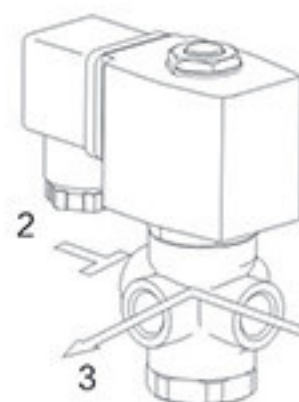
UVMI-A型：常闭型，2为压力供应口
