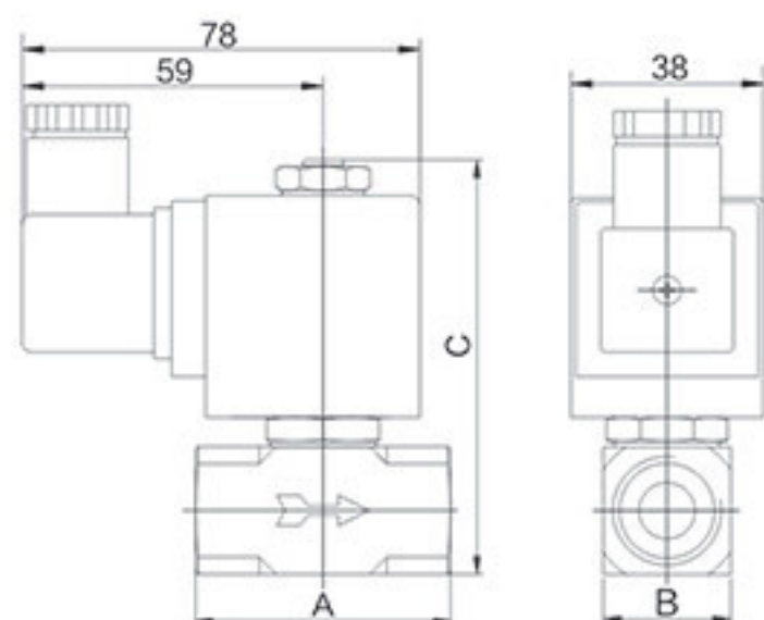
UYSV系列常闭型电磁阀外形图
