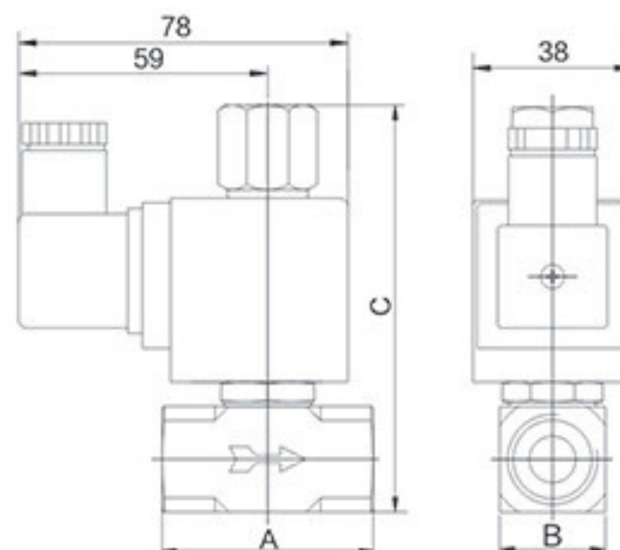
UYSV系列常开型电磁阀外形图
