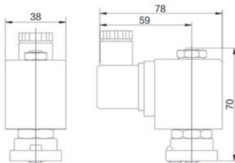
UYSL系列板阀常闭型外形图
