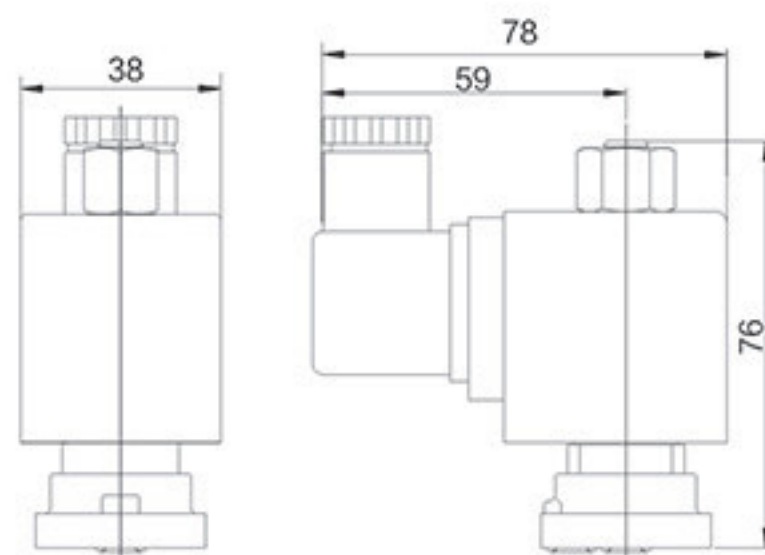
UYSL系列板阀常开型外形图
