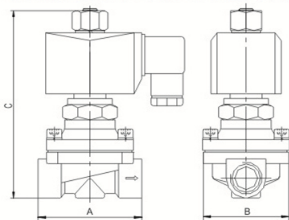
N2W系列分步直动式（常开型）电磁阀外形简图及外形尺寸表
