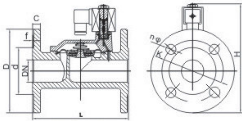
RSP-JF法兰系列外形图
