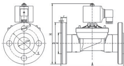
2W-32~50SLF外形图
