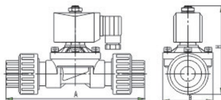
2W-15~25SLH外形图
