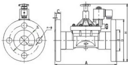
法兰式外形图
