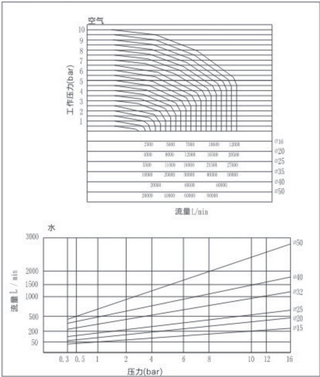
流量曲线图
