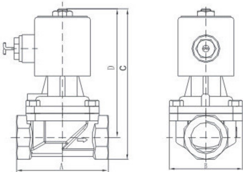
RSPS-15~50螺纹连接系列（常闭型）电磁阀外形图尺寸表
