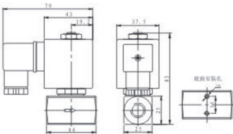
ZCT-3~4N 电磁阀外形图 (适用于通径φ3mm、φ4mm 螺纹 1/8"、1/4")
