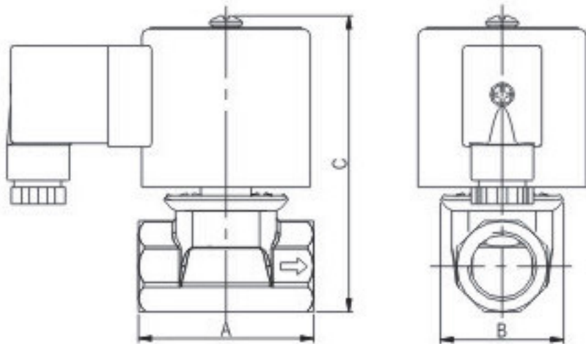
ZCT-6~25电磁阀外形图 (适用于通径φ4.5mm、φ10mm、φ15mm、φ20mm 螺纹 1/4"~1")
