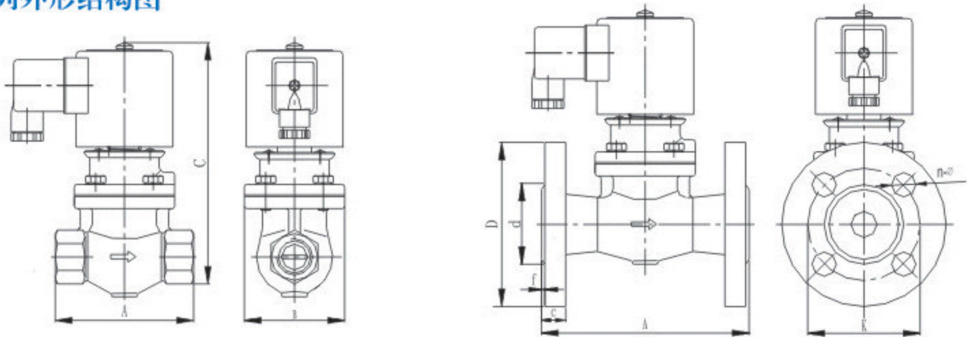
ZCZ-15~50螺纹连接式外形图
