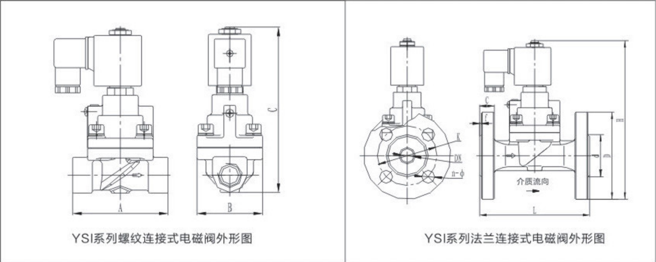
YSI系列螺纹连接和法兰连接式电磁阀外形图
