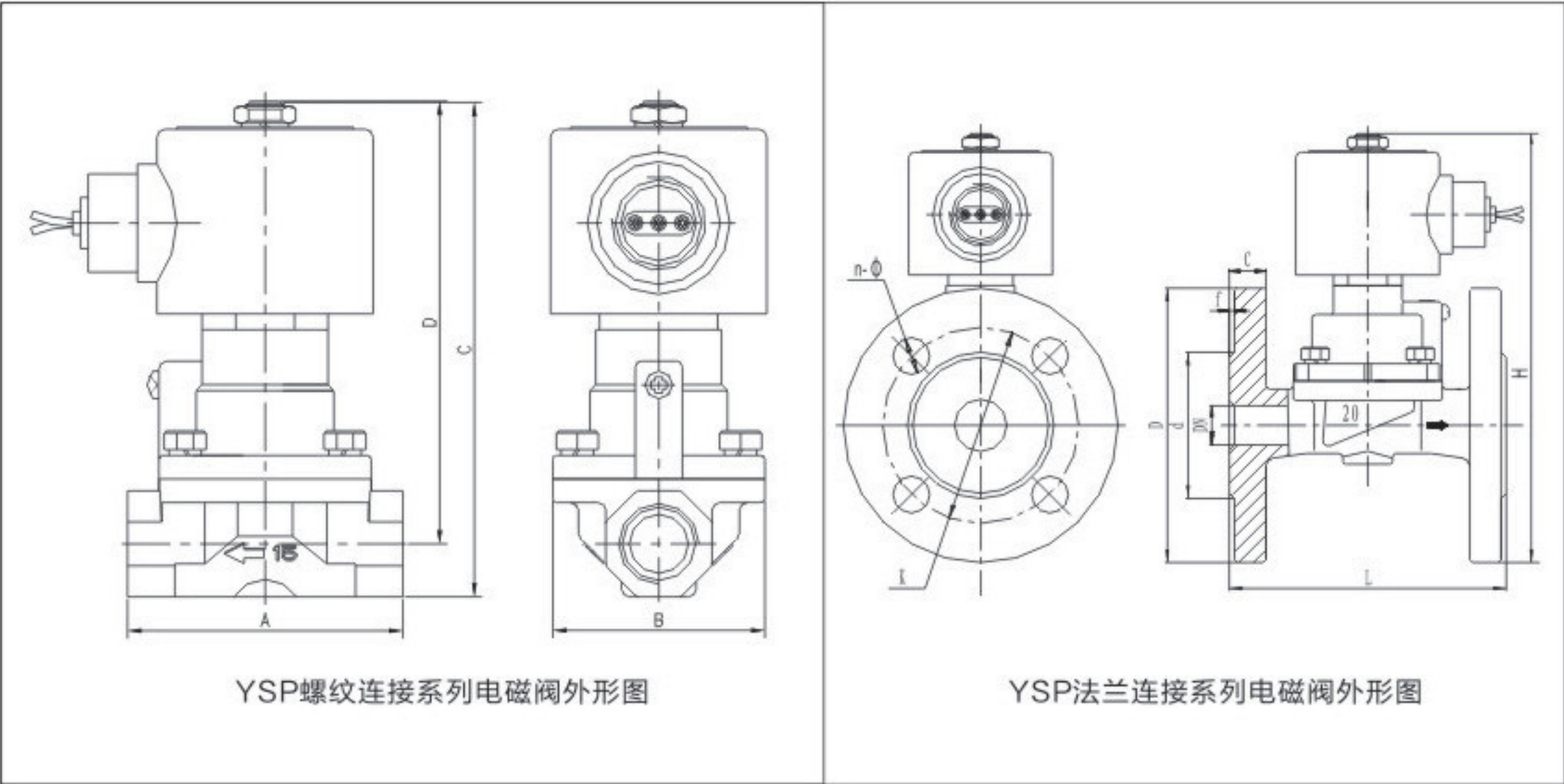
螺纹连接和法兰连接式(常闭型)电磁阀外形图
