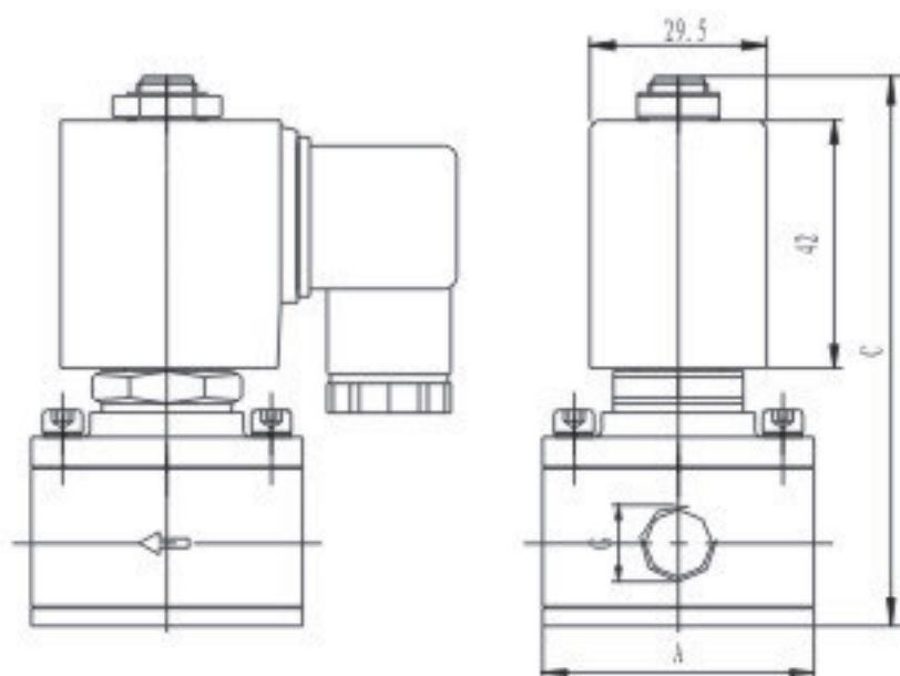
ZCF-2~8外形图
