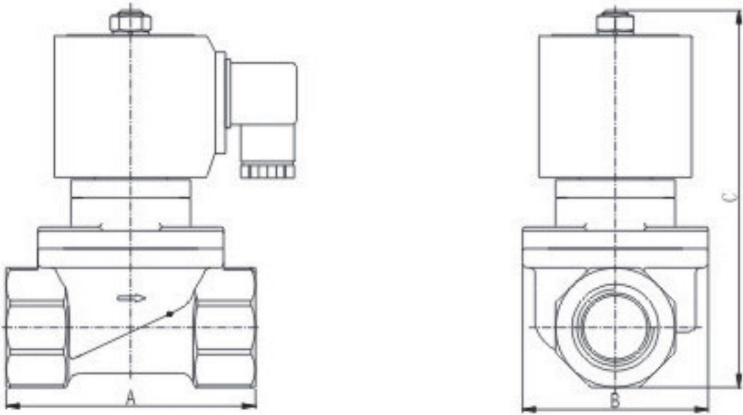
ZCF-P系列防腐电磁阀外形图
