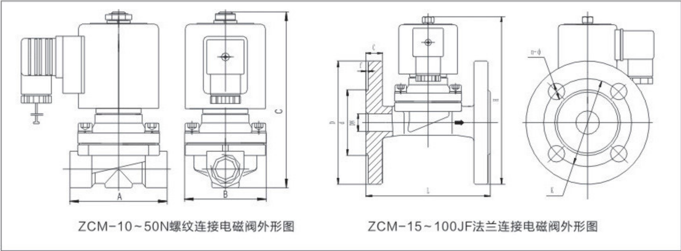
ZCM系列分步直动式煤气电磁阀外形图
