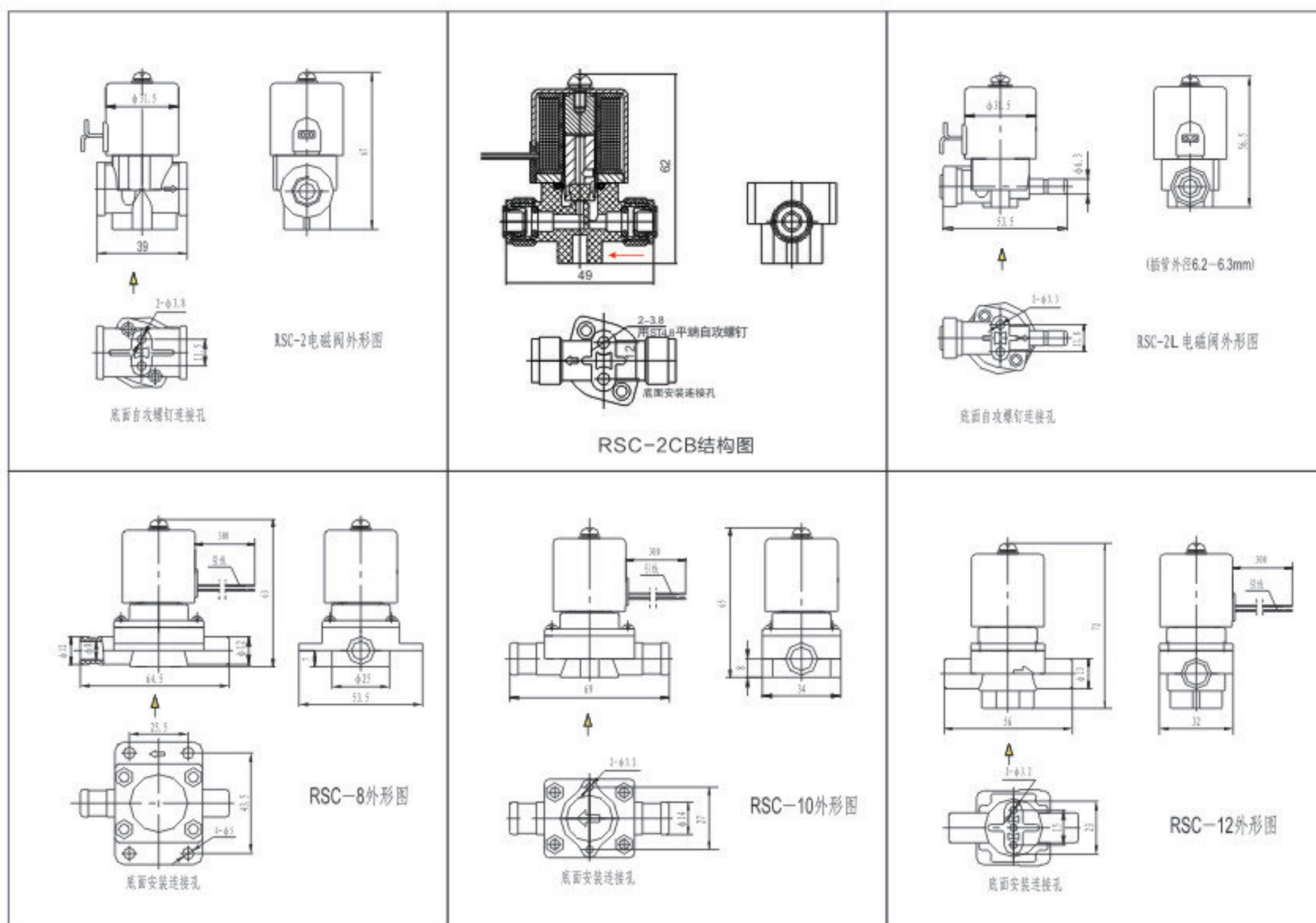
RSC系列电磁阀外形尺寸图
