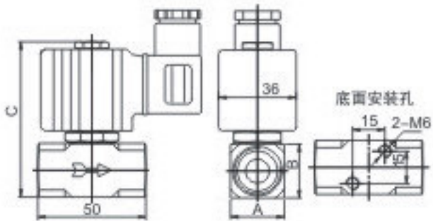
YSV系列外形图
