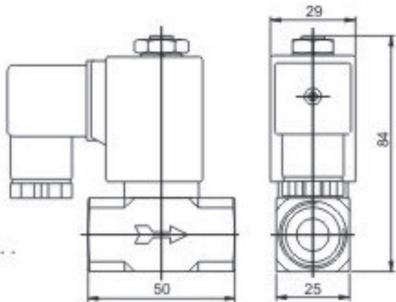
YSV-K系列外形图
