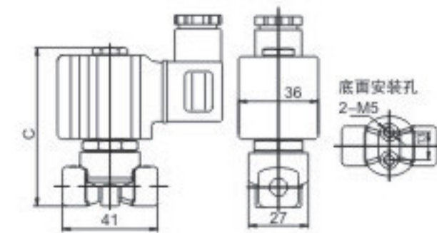
VX2系列外形图
