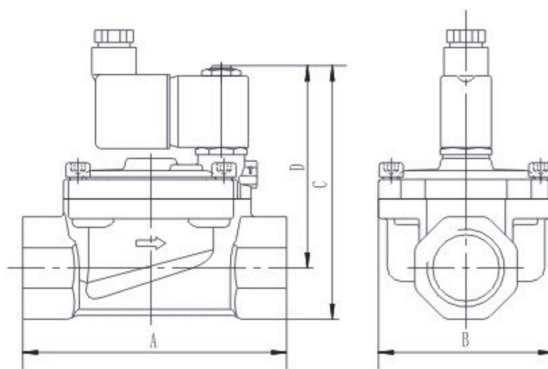
RSQ系列电磁阀外形图
