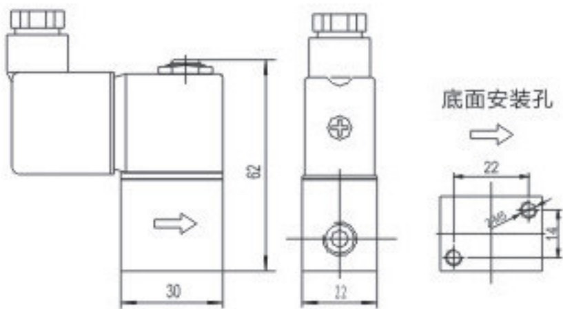
RSV-025-08直动式外形图
