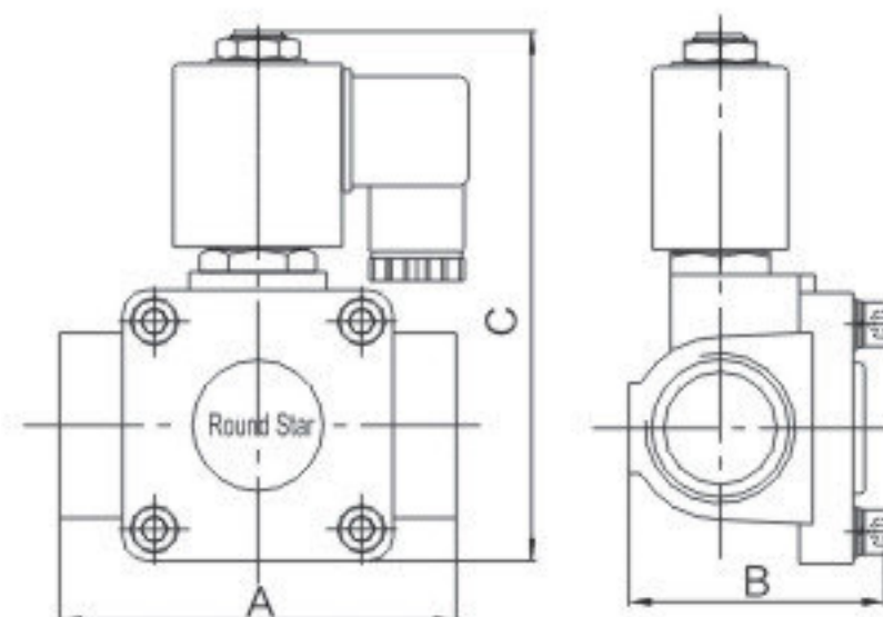
0927系列电磁阀外形简图
