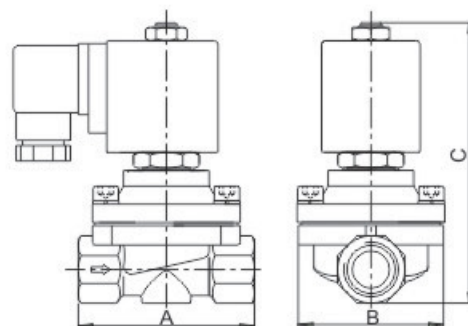
ZK-15~50外形图
