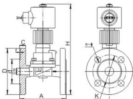
DW系列低温电磁阀法兰连接电磁阀外形图
