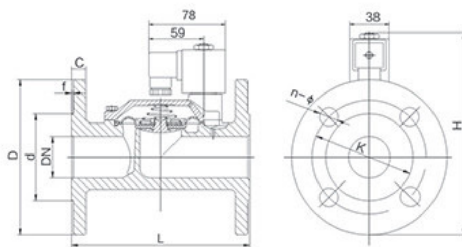
法兰系列外形图
